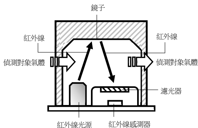
&lt;構造圖&gt;
