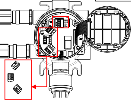
接點輸出用端子台
